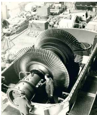
Parní turbína. | Foto: Archiv PBS
