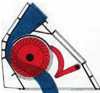
Princip Bánkiho turbíny. | Foto: Zdroj wikipediae
